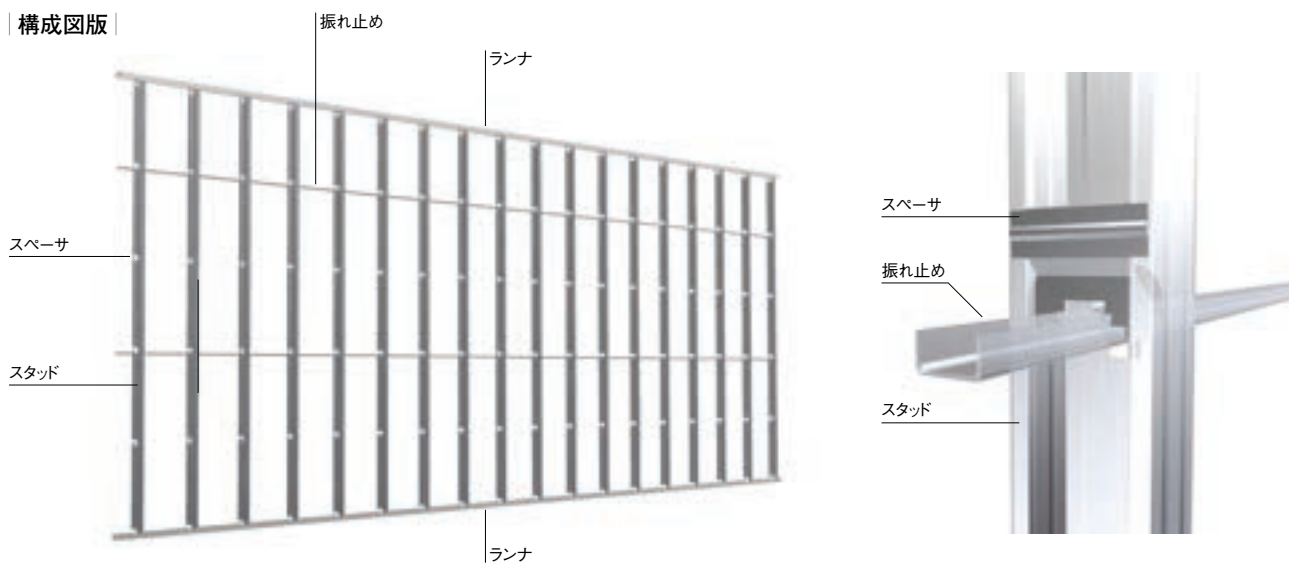
[ 部材一覧 ]
