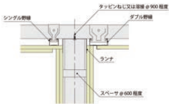
頭部 ランナが野縁と平行の場合
