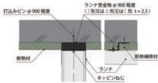
頭部 断熱材ありの場合の取合い
