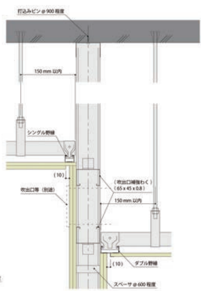
頭部 2室の天井高が異なる場合
