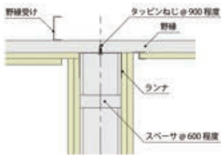
頭部 ランナが野縁と直角の場合
