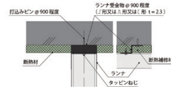
頭部 断熱材ありの場合の取合い
