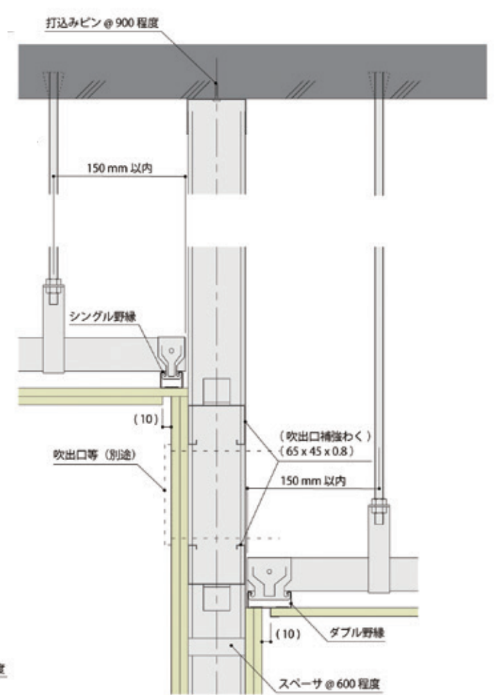
頭部 2室の天井高が異なる場合
