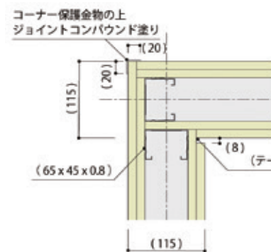
L形取合い
