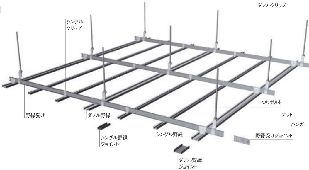
構成図例
