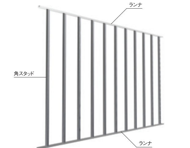
部材一覧 (角スタッド・ランナ)
