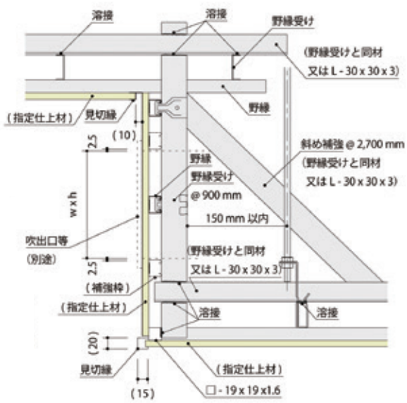
下がり壁と野縁が直角の場合
