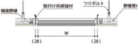
B-B断面
