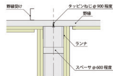
頭部 ランナが野縁と直角の場合
