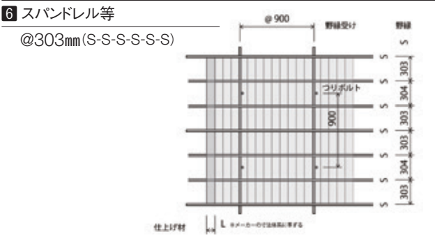
スパンドレル等を下地に張る場合
