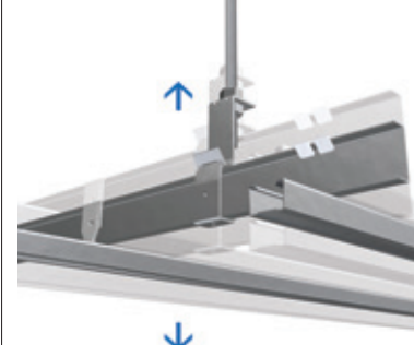
天井高、水平などを調整し、ハンガを固定する
