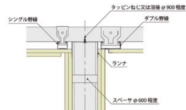
頭部 ランナが野縁と平行の場合
