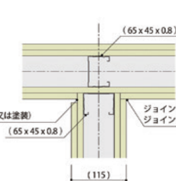
T形取合い
