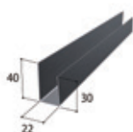
ランナ20L
