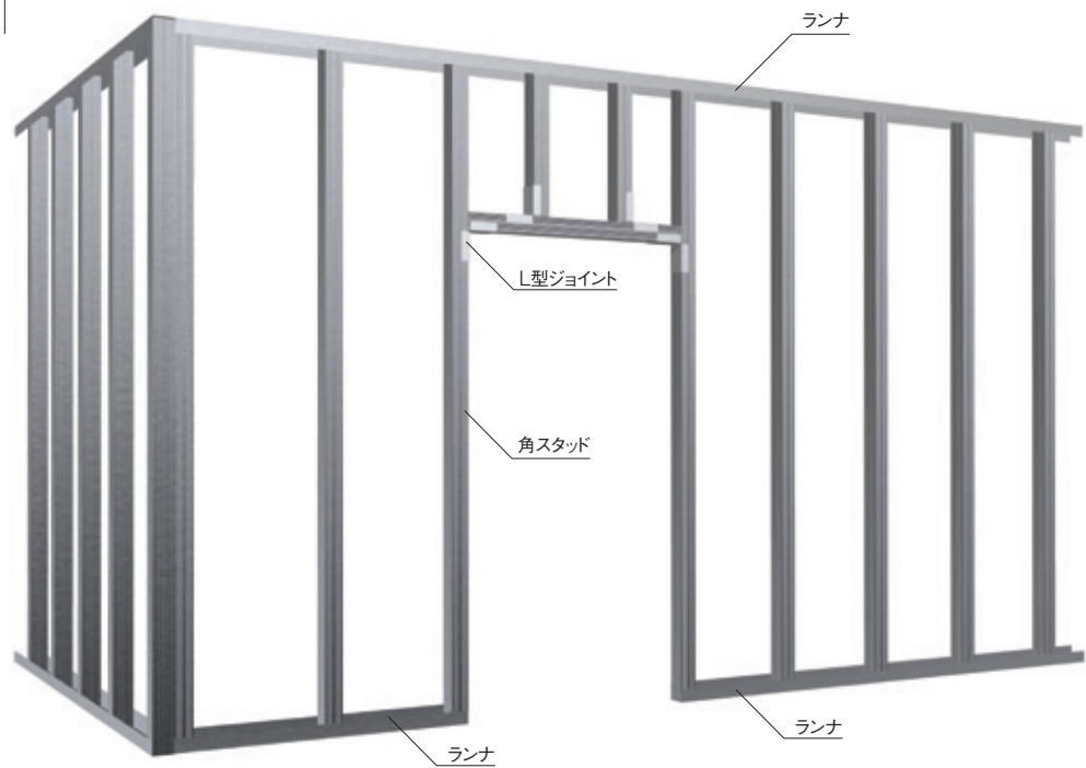
間仕切り壁
