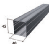
角スタッド4045
