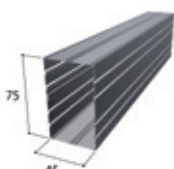
角スタッド4575
