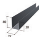
ランナ25L
