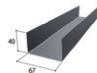
ランナ65L
