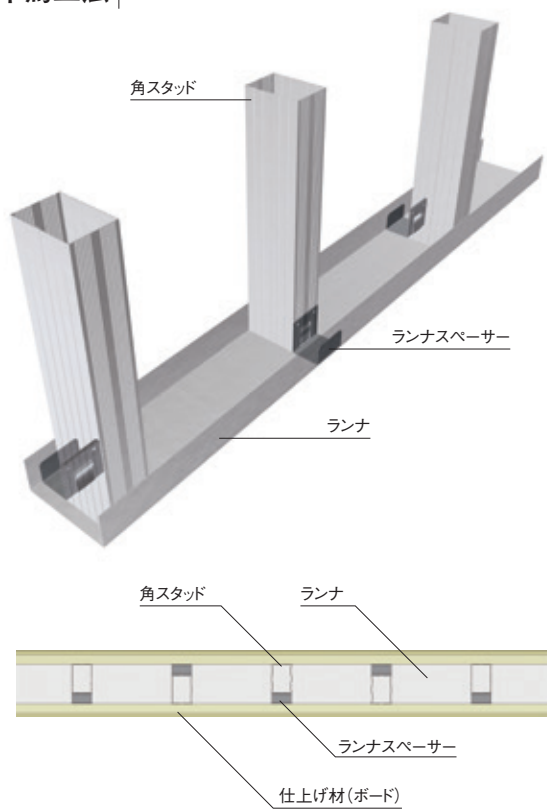
千鳥工法
