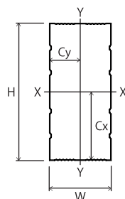
角スタッド
