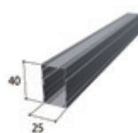
角スタッド4025
