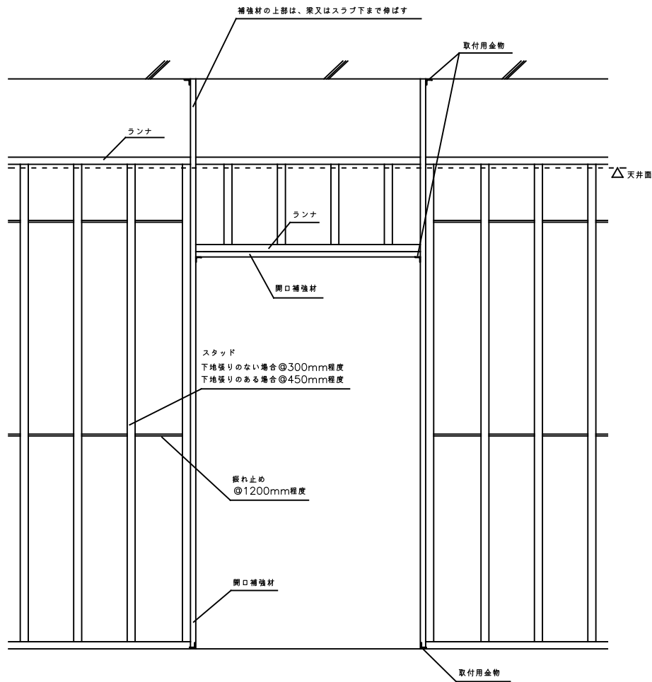
上部ランナを鋼製天井下地に固定する場合
