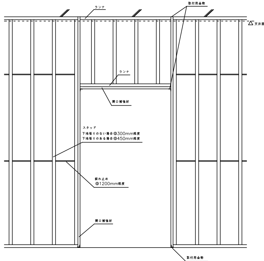
上部ランナをスラブ下に固定する場合
