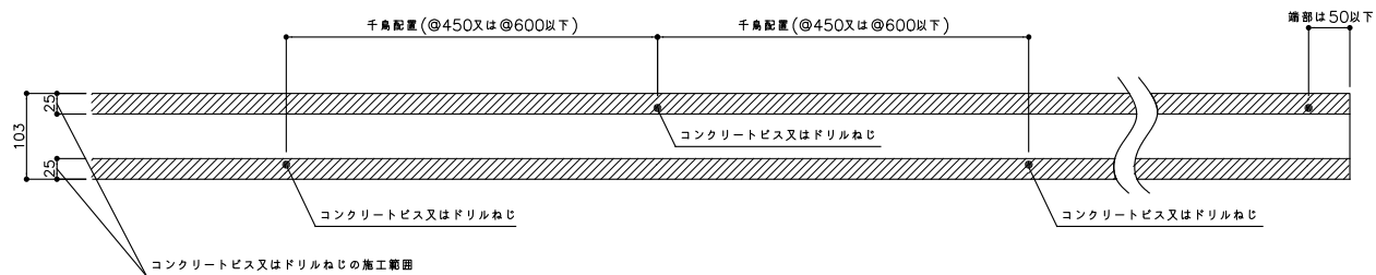
コンクリートビスおよびドリルねじの配置と施工範囲(単位:mm)
