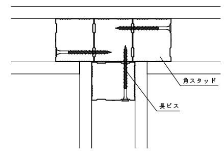
T字コーナー
