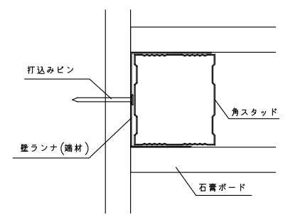
A-A 断面
