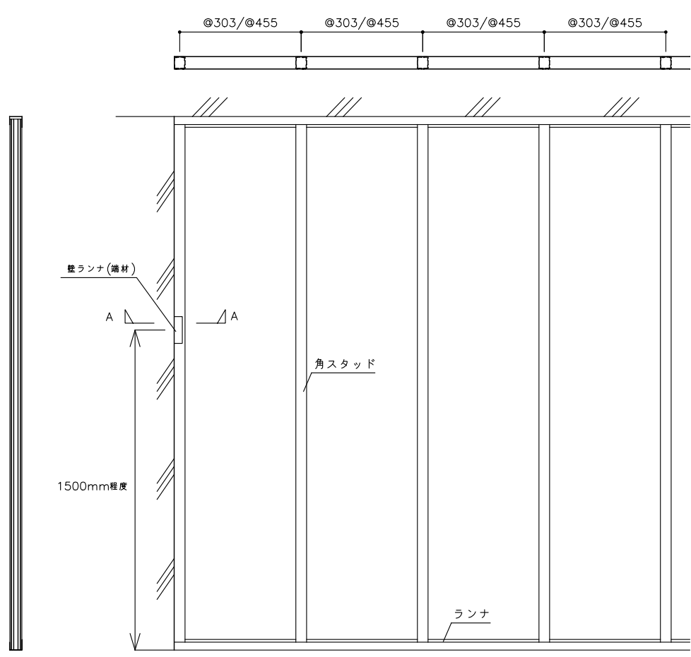
端部納まり
