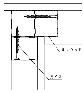
L字コーナー
