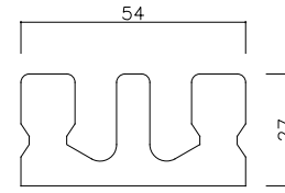
シダブルクリップ：SUSクリップW25
