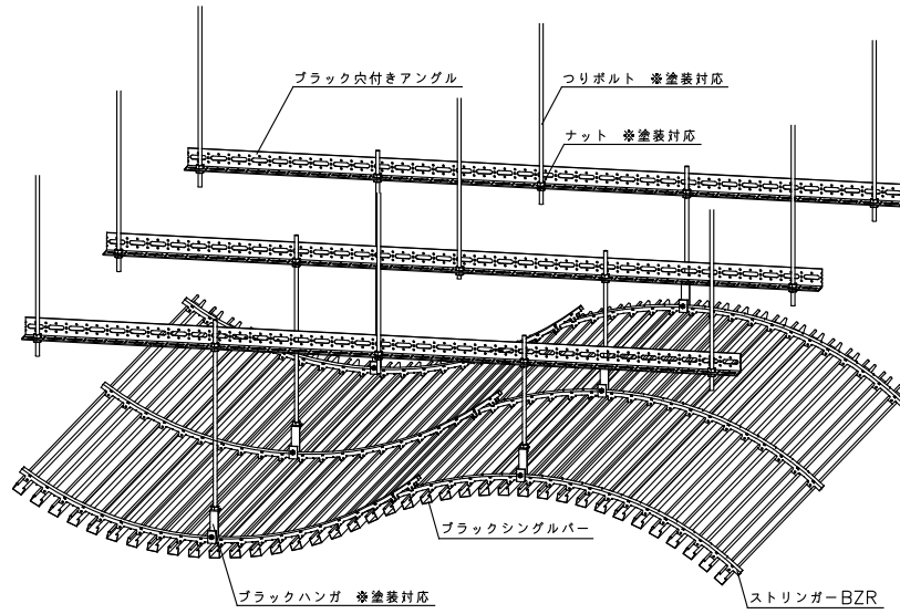
構成図例
