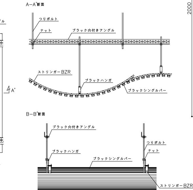
断面図
