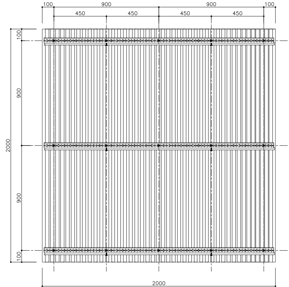
納まり図例
