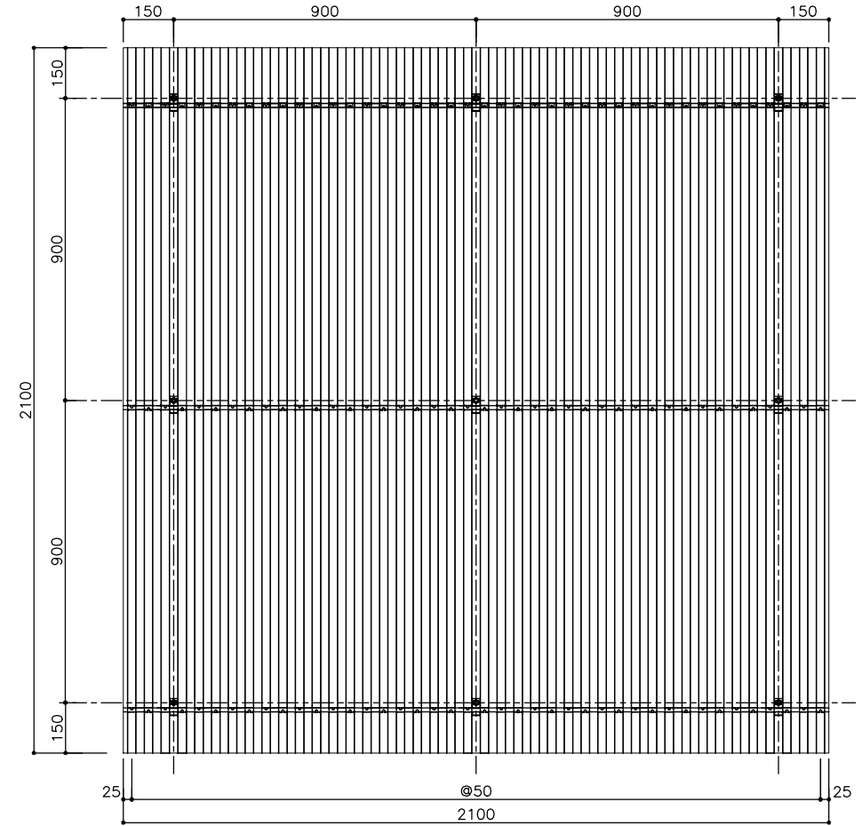
納まり図例
