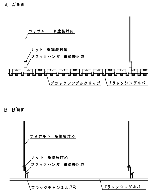
断面図
